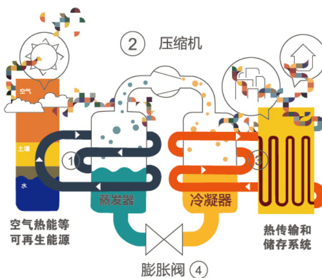
图1-3 热泵技术原理图
