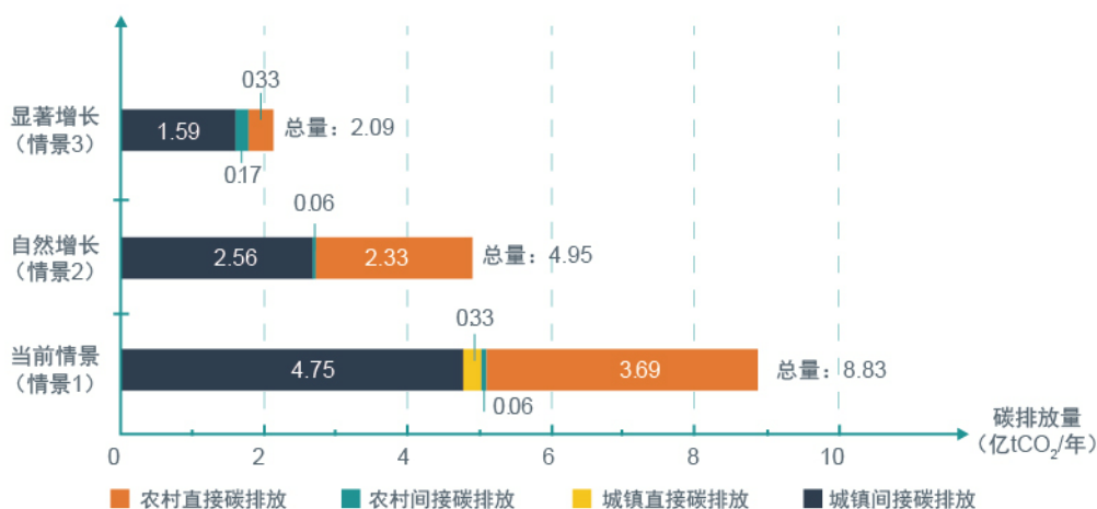
图5-5 建筑供暖不同情景下的碳排放
