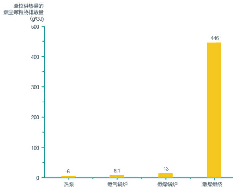
图5-31 不同供热方式单位供热量的烟尘颗粒物排放量
