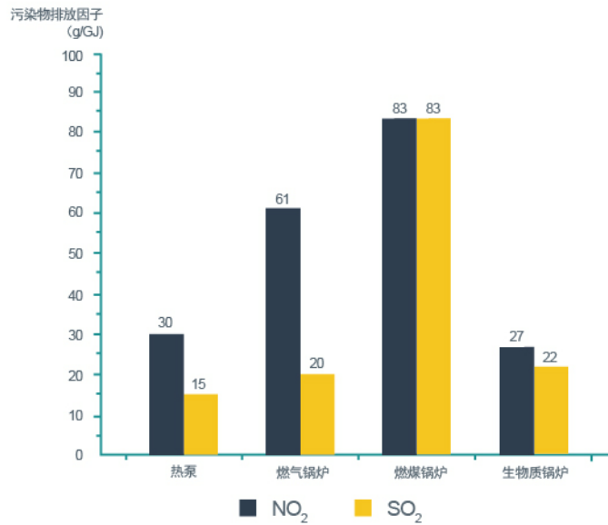
图5-30 不同供热方式单位供热量的污染物排放因子
