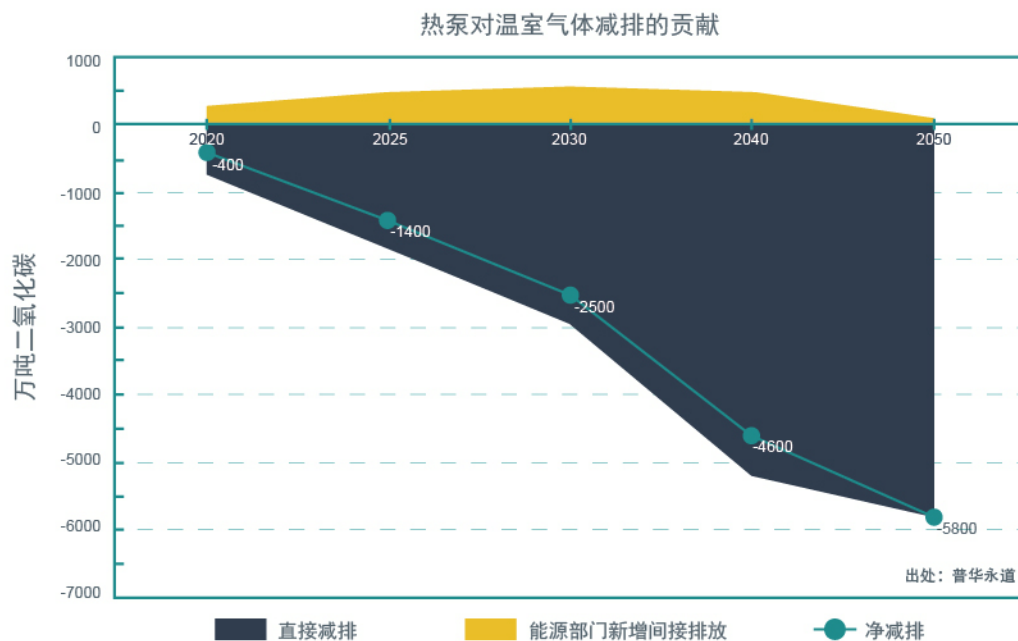
图4-10 热泵在在供暖领域的减排潜力
