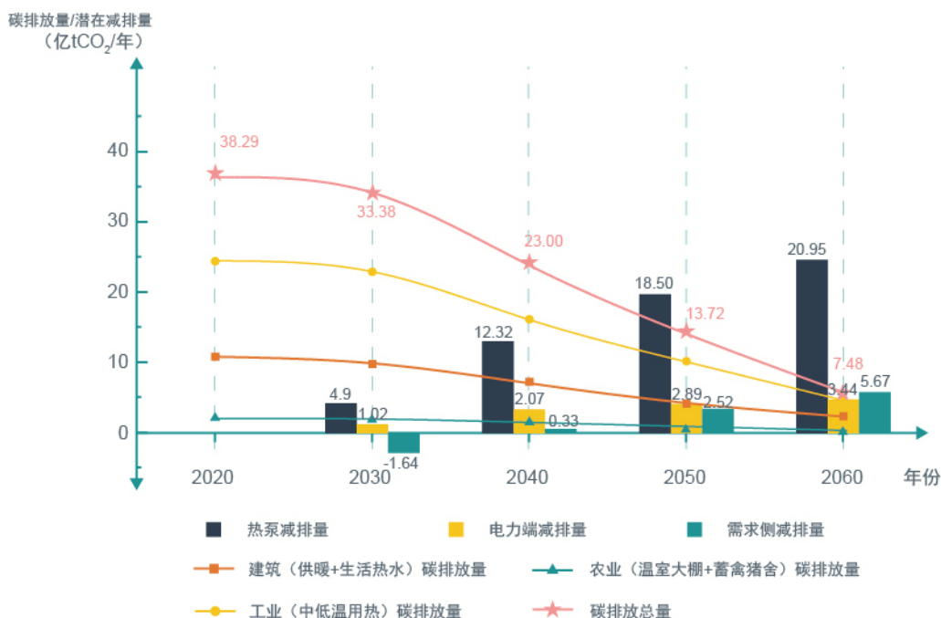
图5-26 碳排放总量逐年变化
