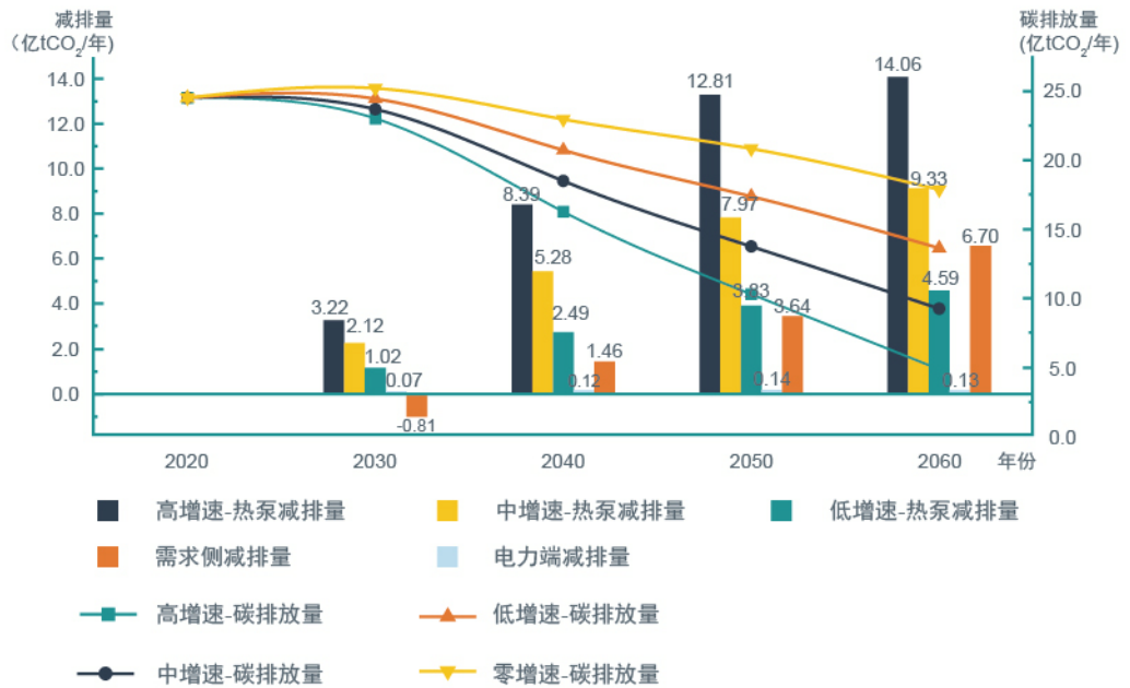
图5-13 工业生产不同热泵增速下的碳排放量与减排量
