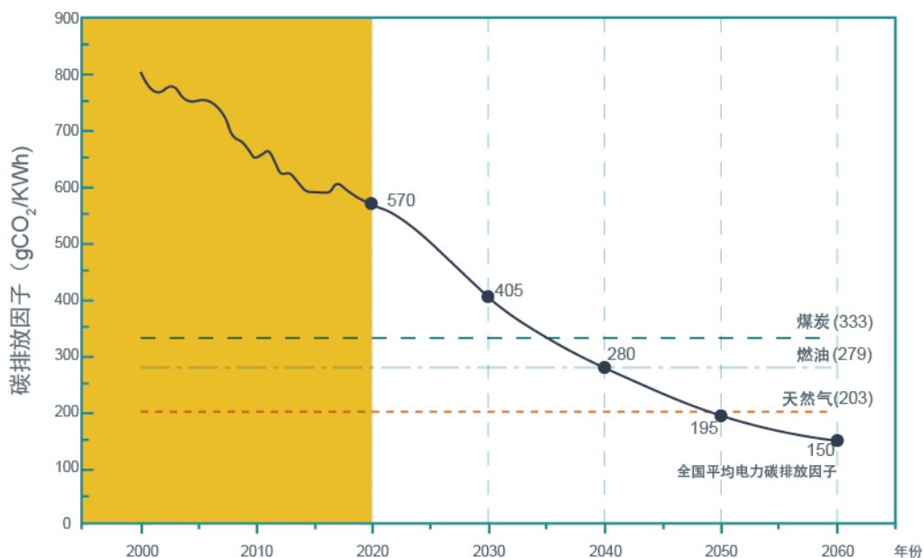
图5-1 相关能源的碳排放因子
