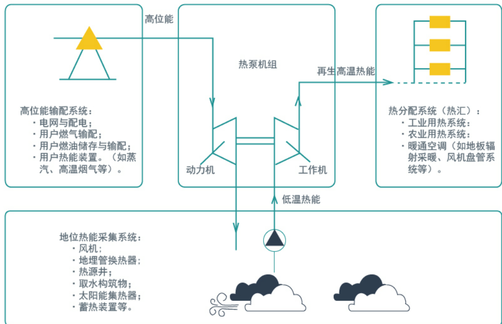
图2-2 热泵系统
