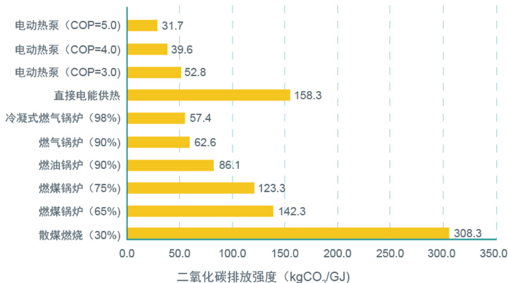
图4-2 不同供热系统的碳排放强度
