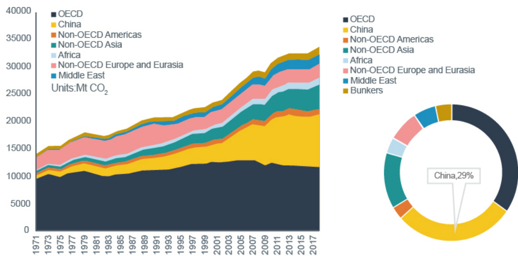
图1-1 1971-2018年世界燃料燃烧产生的二氧化碳排放量及占比
