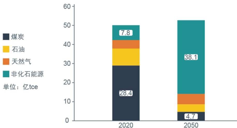
图1-2 2°C情景下分品种的能源消费构成
