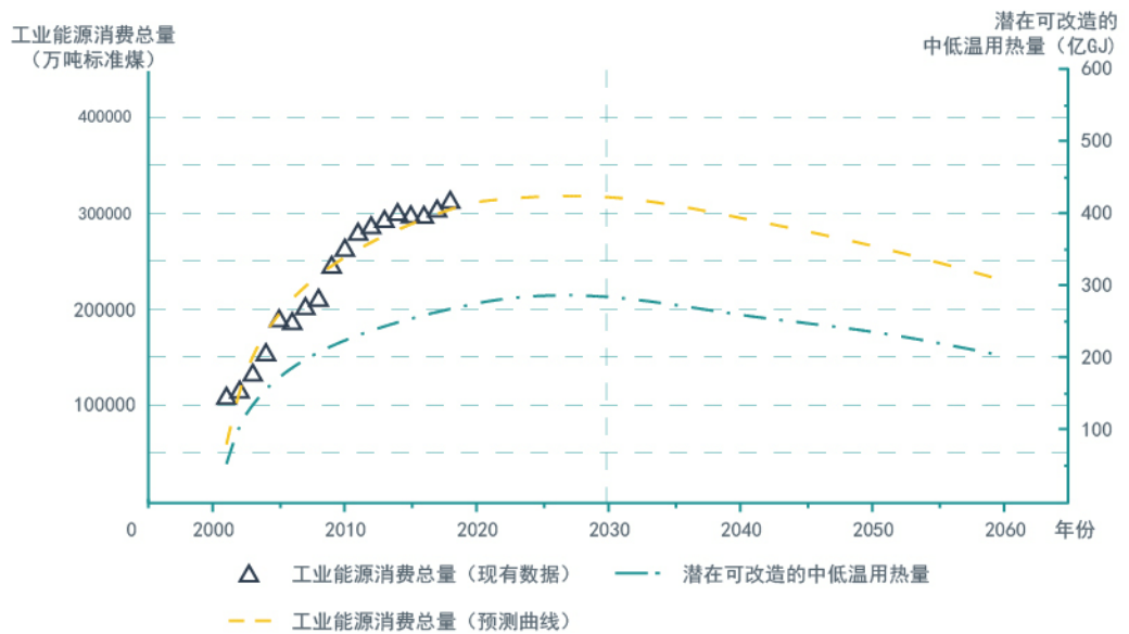
图5-11 工业能源与用热量预测
