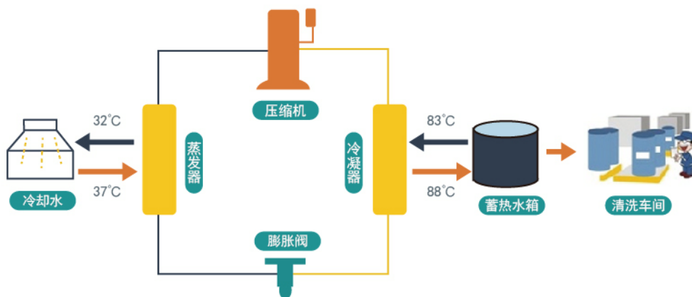
图4-6 酸奶厂应用热泵流程
