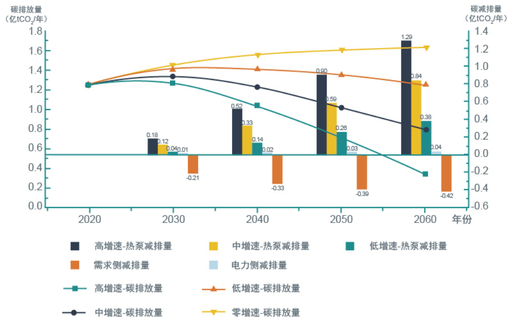
图5-17 农业大棚不同热泵增速下的碳排放量与减排量
