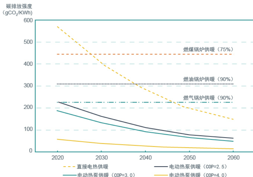
图5-7 采用不同热源供暖的碳排放强度变化
