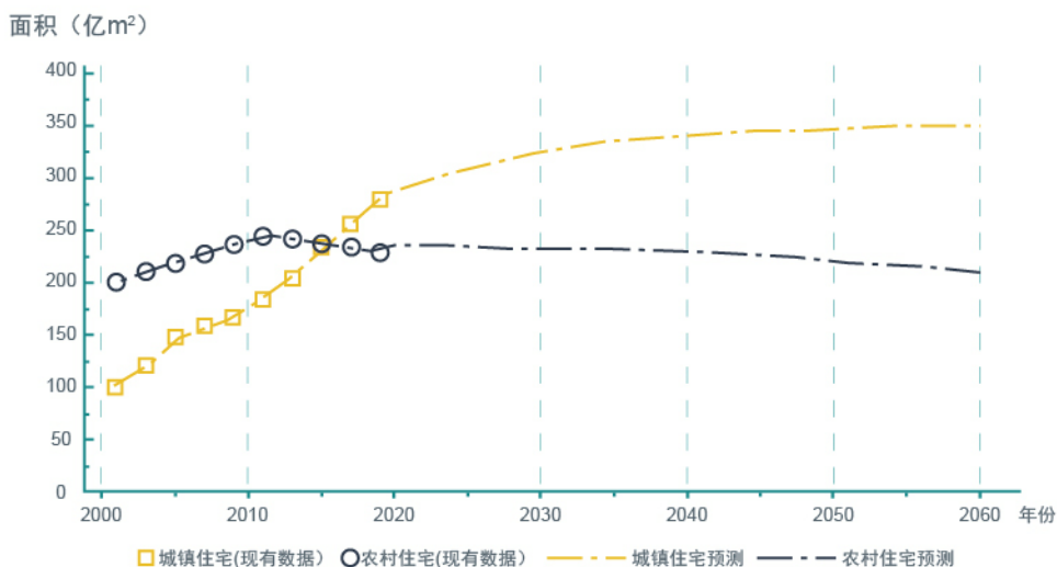
图5-3 城镇和农村住宅规模预测
