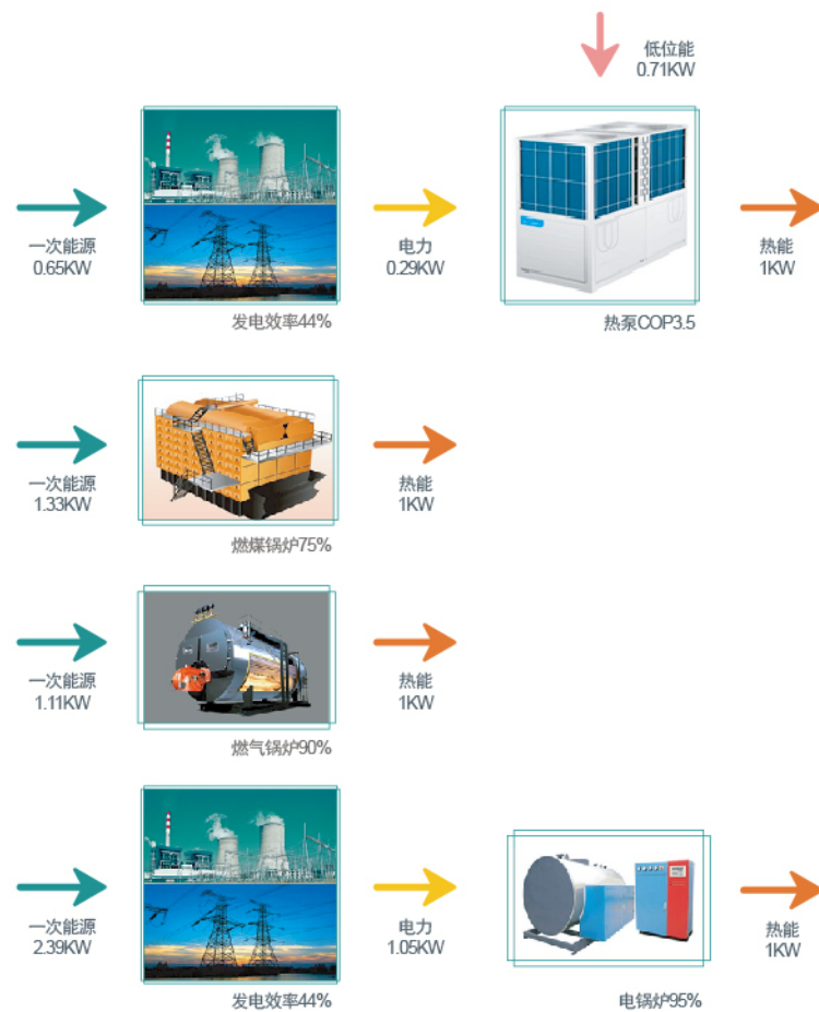
图5-32 不同供热方式一次能源消耗对比
