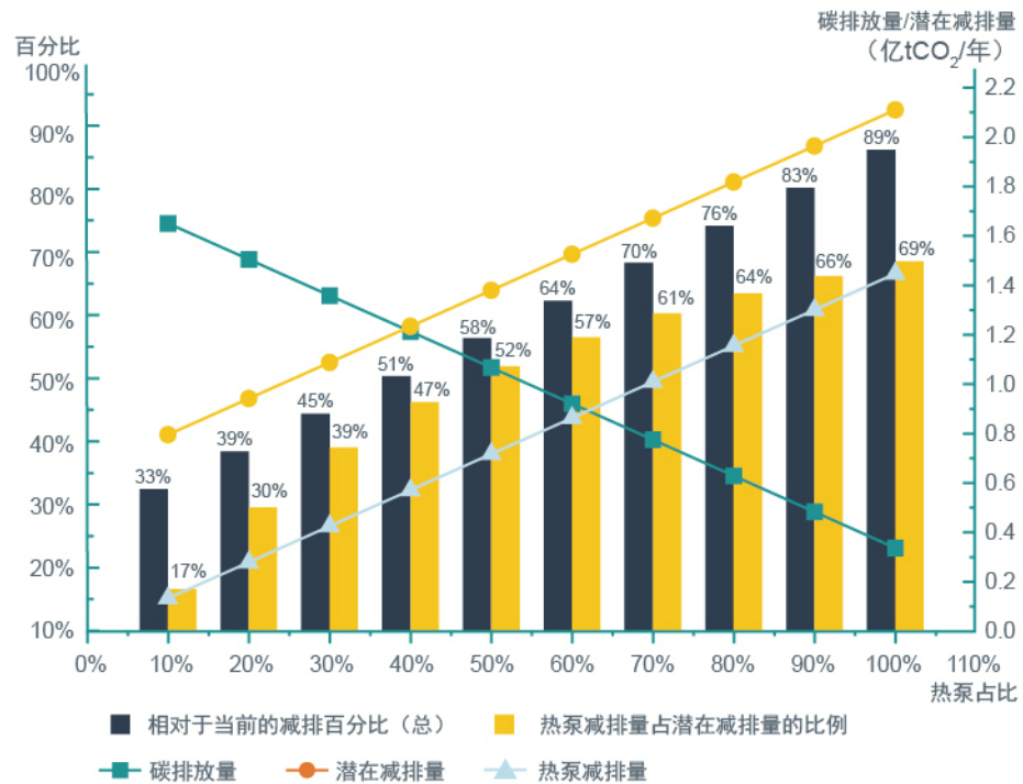
图5-14 2060年工业生产碳排放量、减排量随热泵占比的变化
