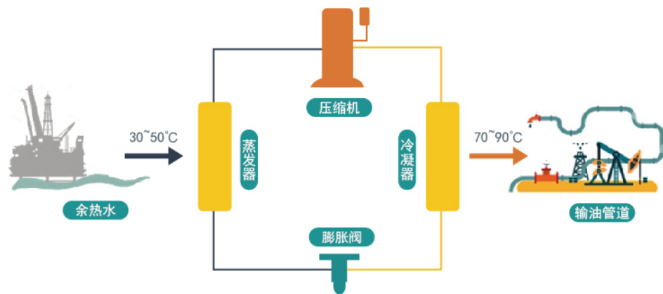
图4-5 原油集输系统加热工艺流
