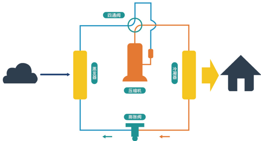
图2-3 空气源热泵
