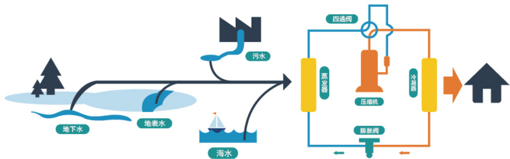
图2-5 水源热泵
