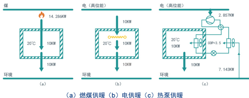
图2-1 不同供暖方案
