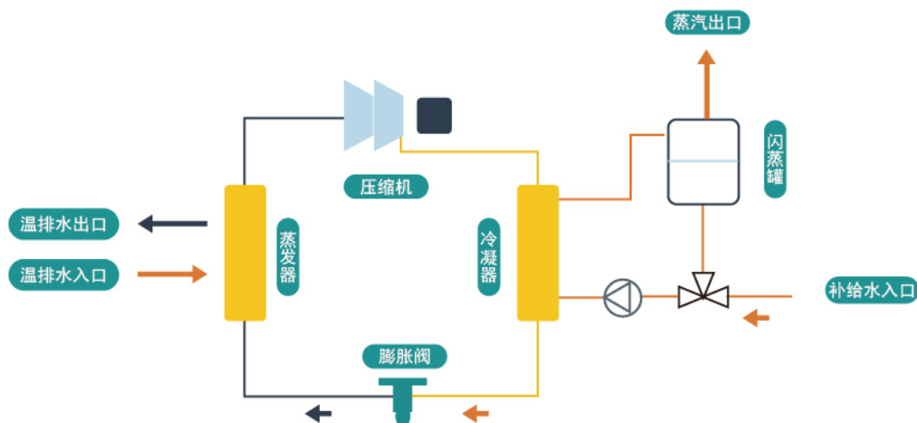
图4-4 SGH120 蒸汽热泵系统流程图
