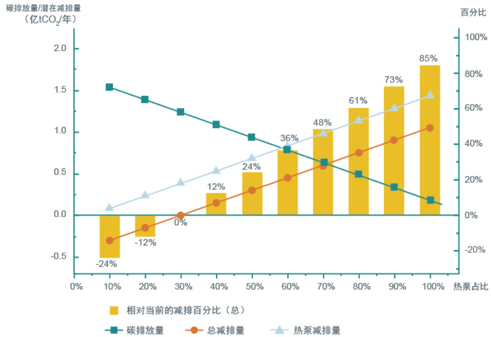
图5-18 2060年温室大棚碳排放量、减排量随热泵占比的变化
