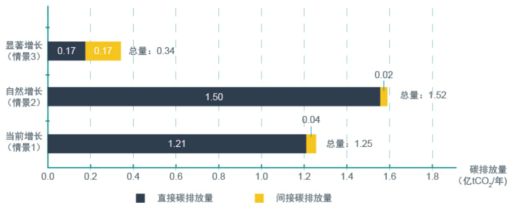
图5-16 温室大棚不同情景下2060年碳排放
