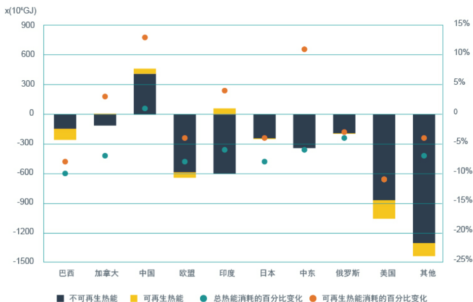
图3-7 2020年部分地区工业用热量同比变化
