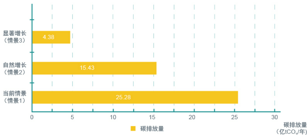
图5-12 工业生产不同情景下的碳排放
