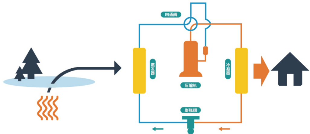
图2-4 土壤源热泵
