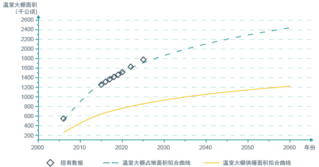
图5-15 我国温室大棚面积趋势预测
