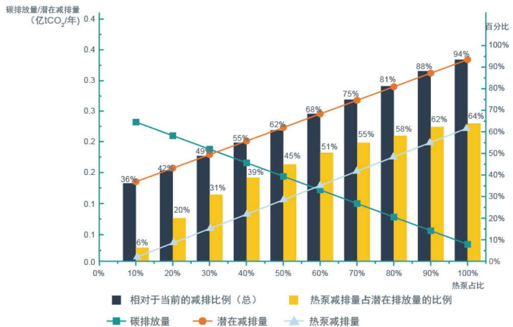
图5-22 2060年畜禽养殖碳排放量、减排量随热泵百分比变化
